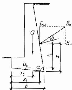
图 6.7.5-2 挡土墙抗倾覆稳定验算示意
