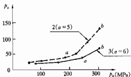
图 8 载荷板压力 p_0 与界面压力 p_z 关系
